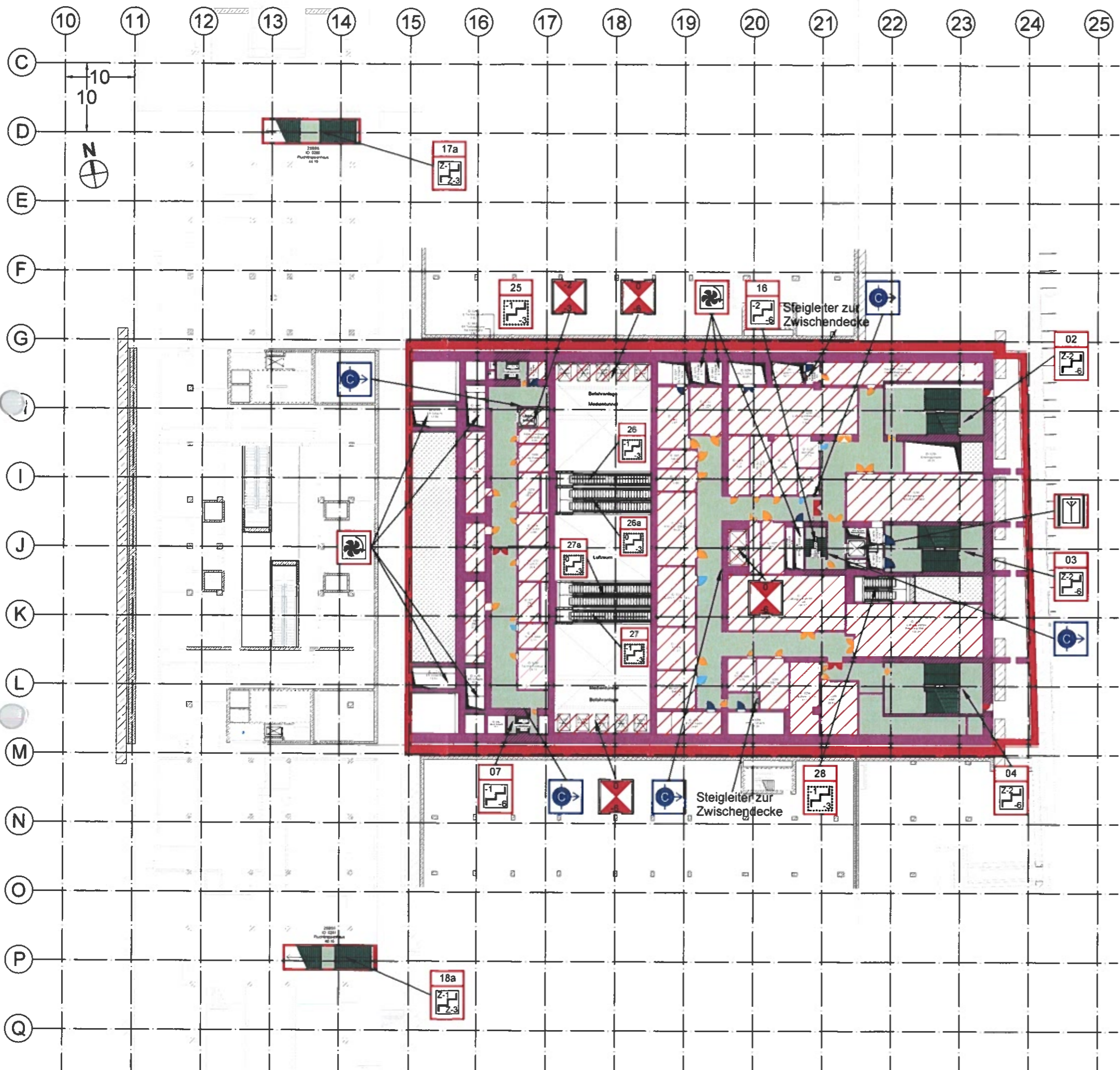
Ebene -2 (Technikgeschoss)
