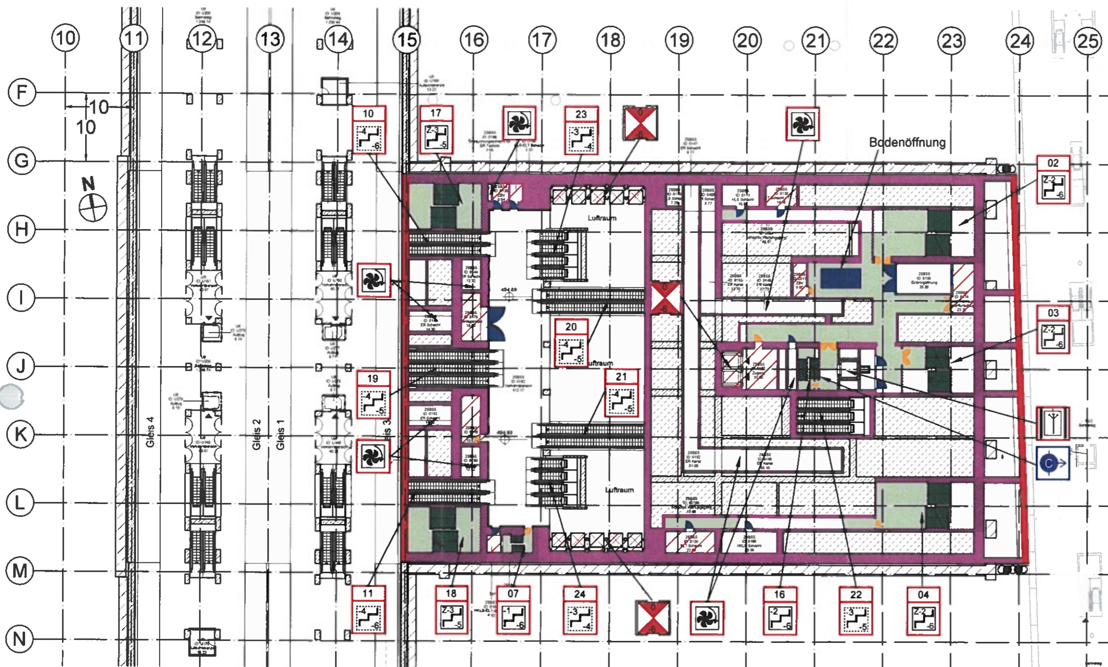
Ebene -4 (Technik-Verteilerebene)
