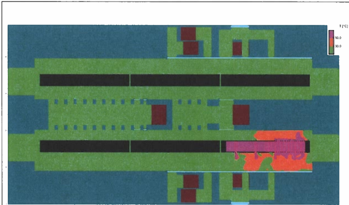
Bild 7: Temperatur in einer Höhe von ca. 1,5 m über der Bahnsteigoberkante 35 Minuten nach Brandbeginn (Grundriss)
