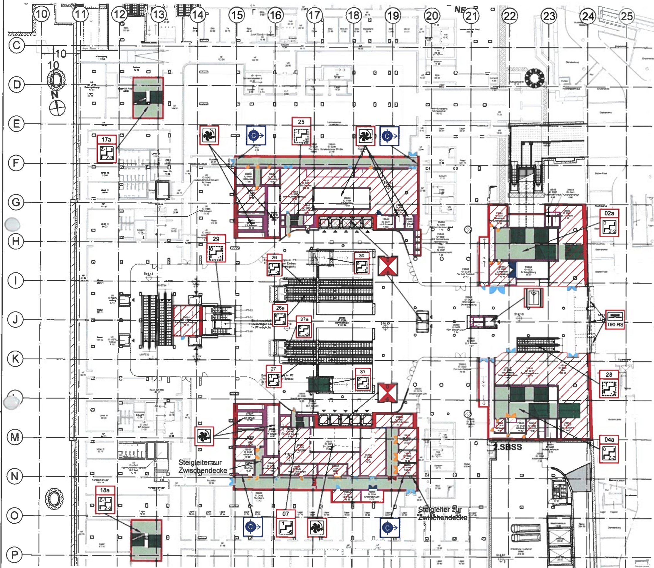
Ebene -1 (Sperrgeschoss)
